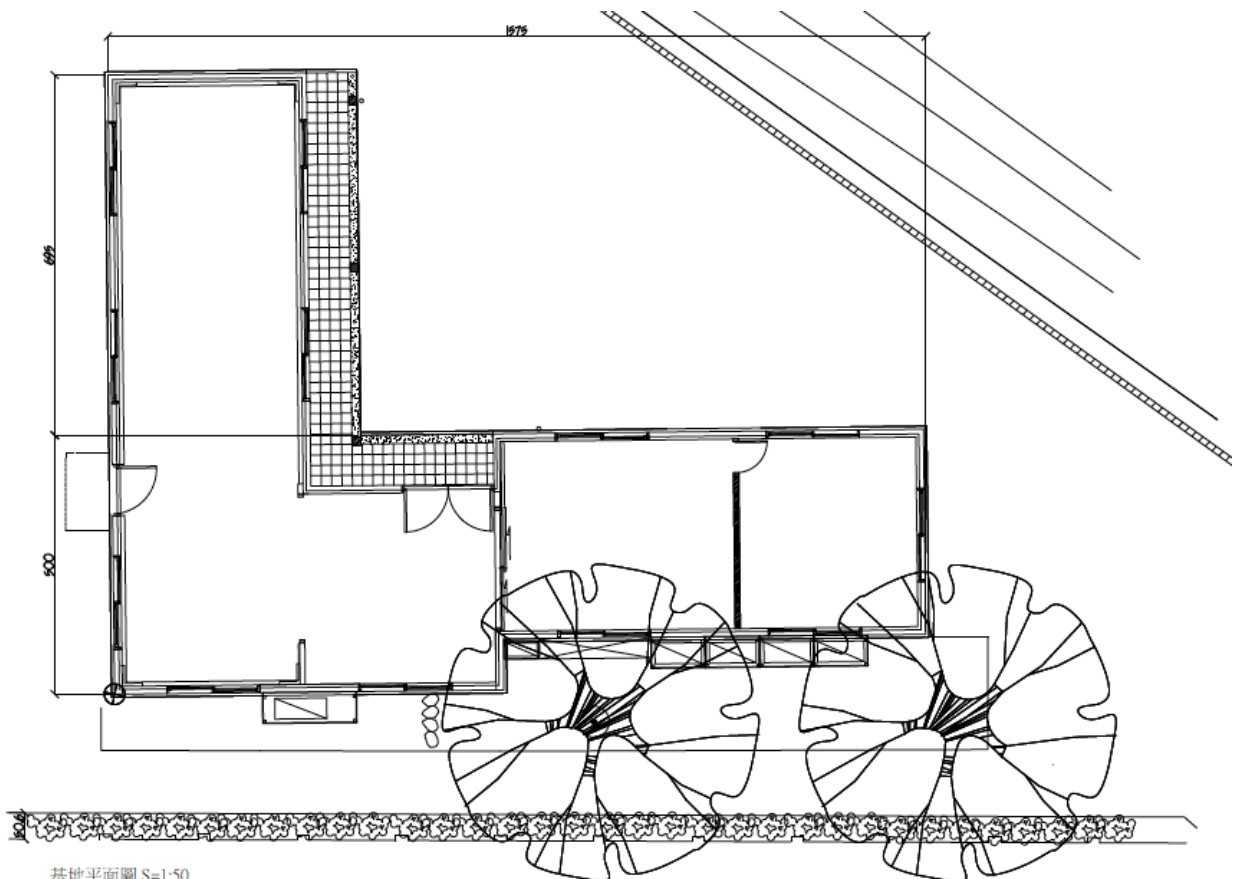
圖 1 基地平面圖
