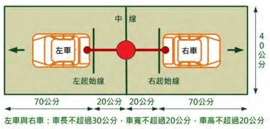
圖5 太陽能車拔河競賽示意圖
