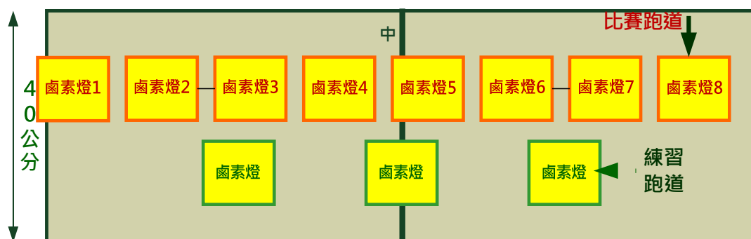
圖4 競賽場地鹵素燈擺放示意圖
